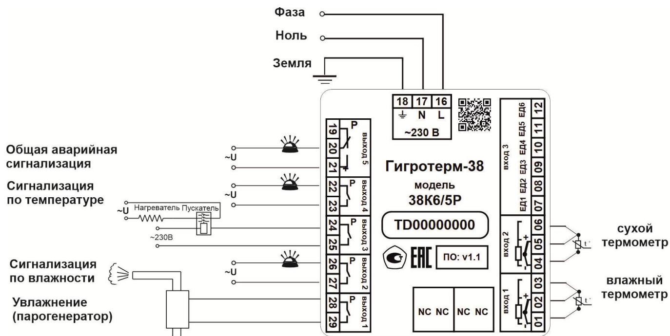
Схема 2. Регулирование влажности с применением парогенератора, регулирование температуры при помощи нагревателя ( N > 1.5 кВт). Для измерения влажности и температуры используется психрометрический метод (сухой и влажный термометры)
