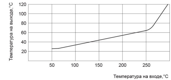
График для отвода-охладителя OC100-OX28
