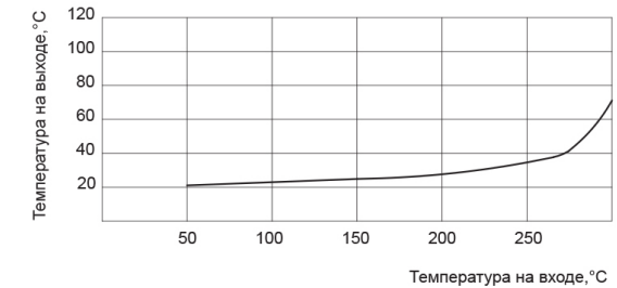
График для отвода-охладителя OC200-OX50
