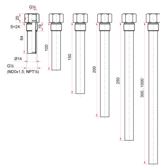
Гильзы из нержавеющей стали (под заказ)
