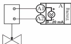
Подключение задвижки с электроприводом
